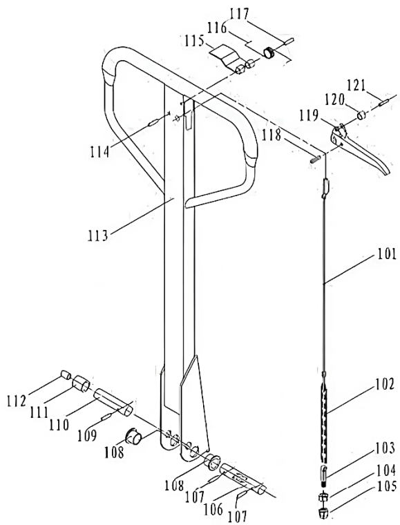
Рисунок 4 – Взрыв-схема ручки тележки АС
