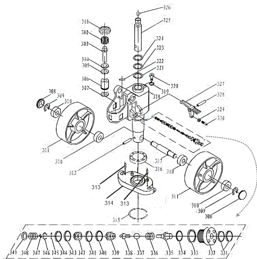
Рисунок 6 – Взрыв-схема гидроузла тележки АС
