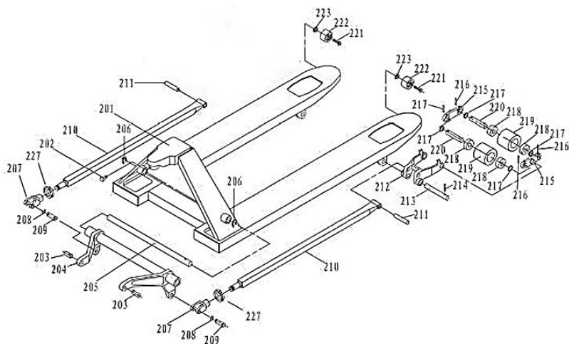
Рисунок 5 – Взрыв-схема корпуса тележки АС
