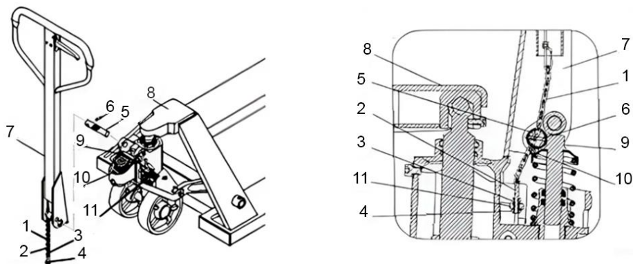
Рисунок 2 – Установка ручки
